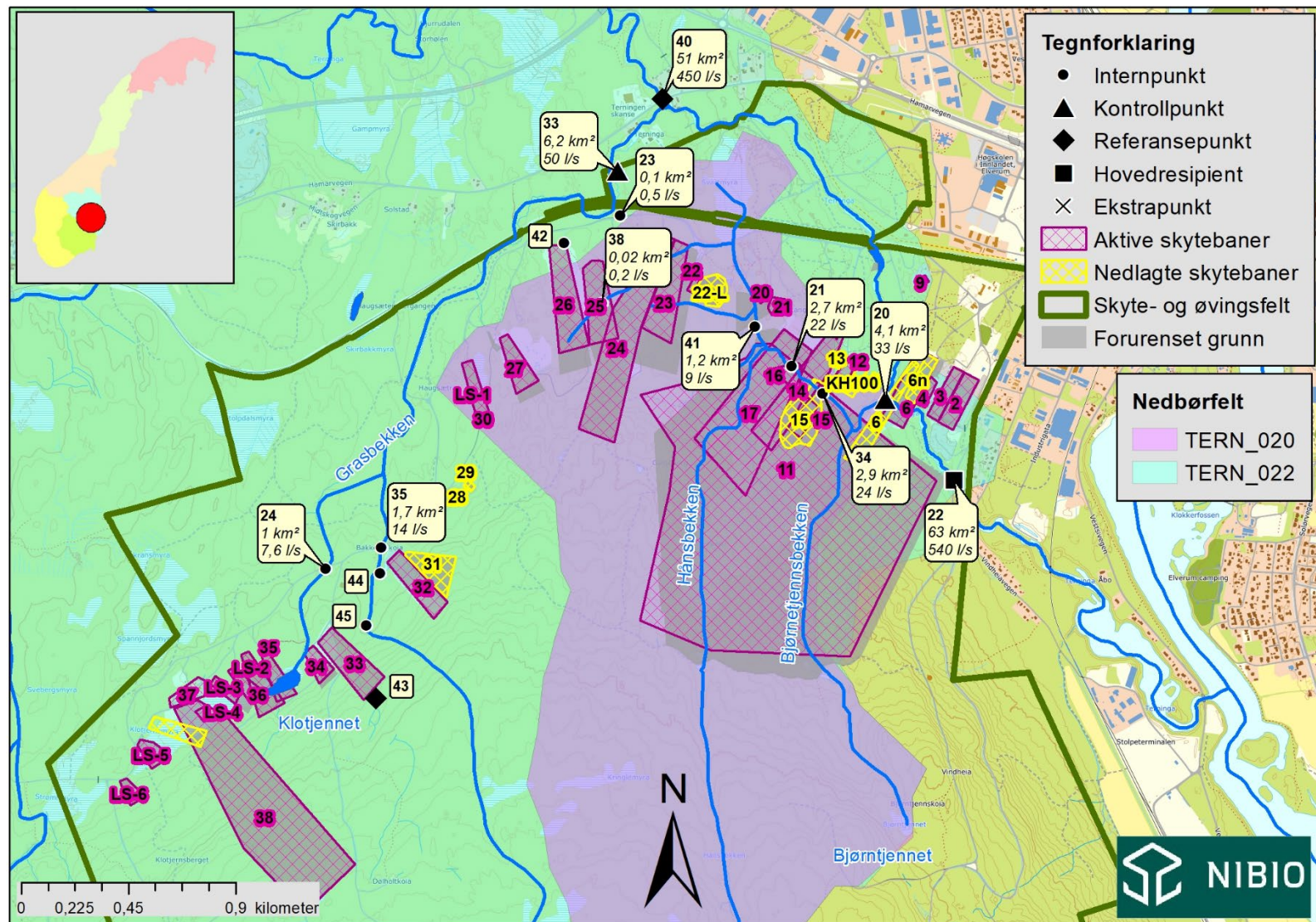
Figur 1. Prøvepunkter med delnedbørfelt på Terningmoen SØF i 2020.
